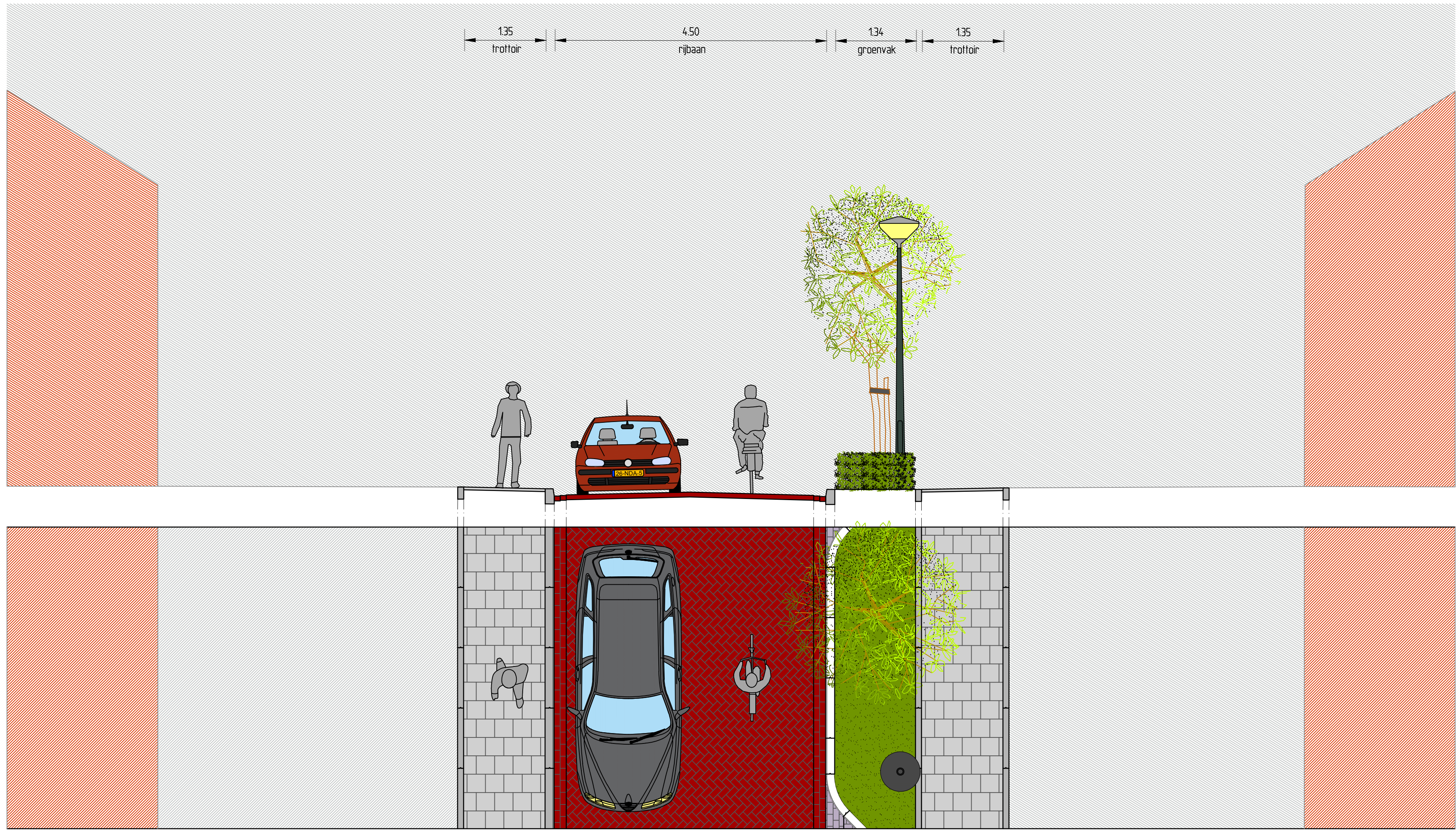
Dwarsprofiel A-A schaal: 1 : 50
