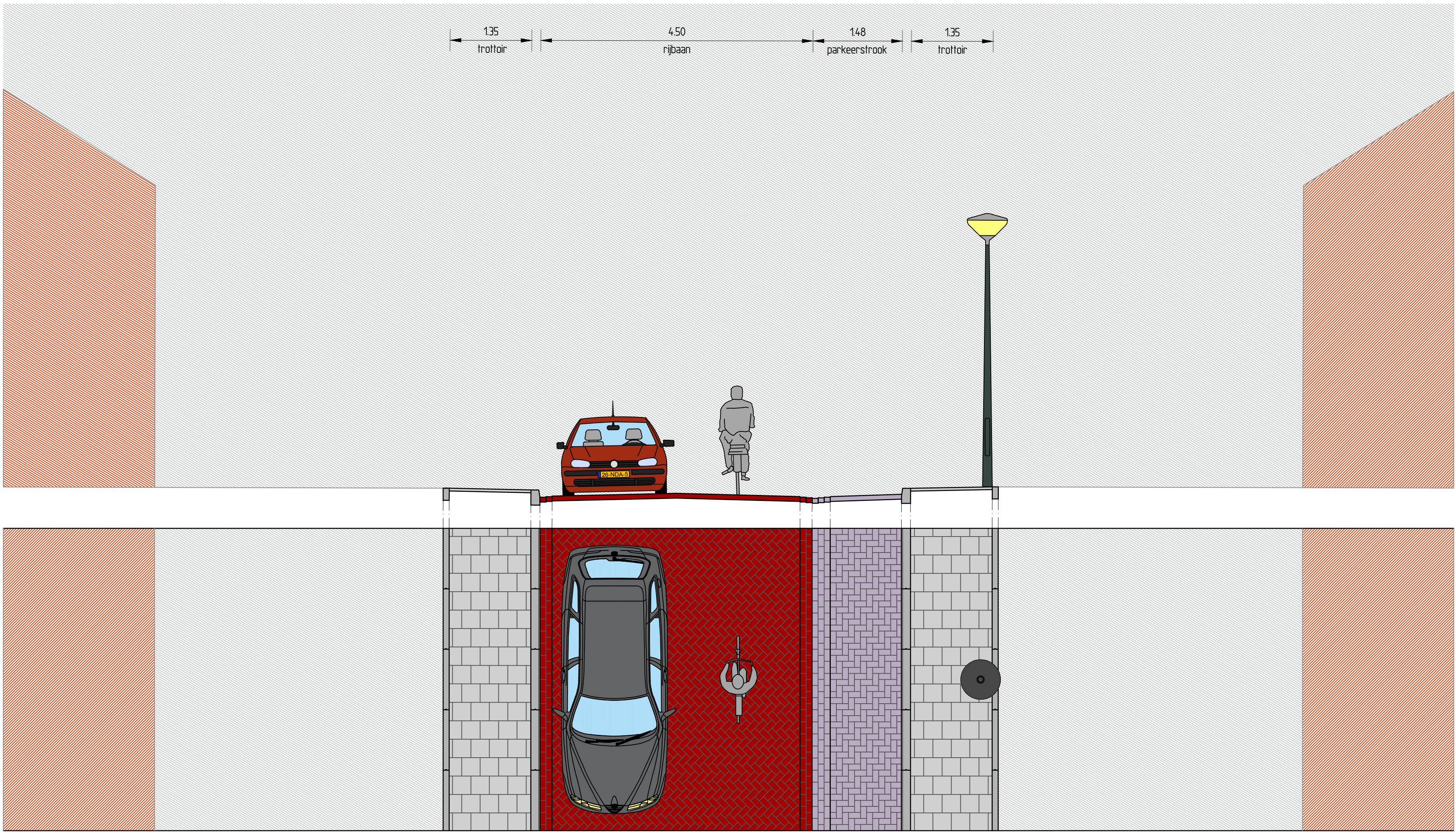
Dwarsprofiel B-B schaal: 1 : 50
