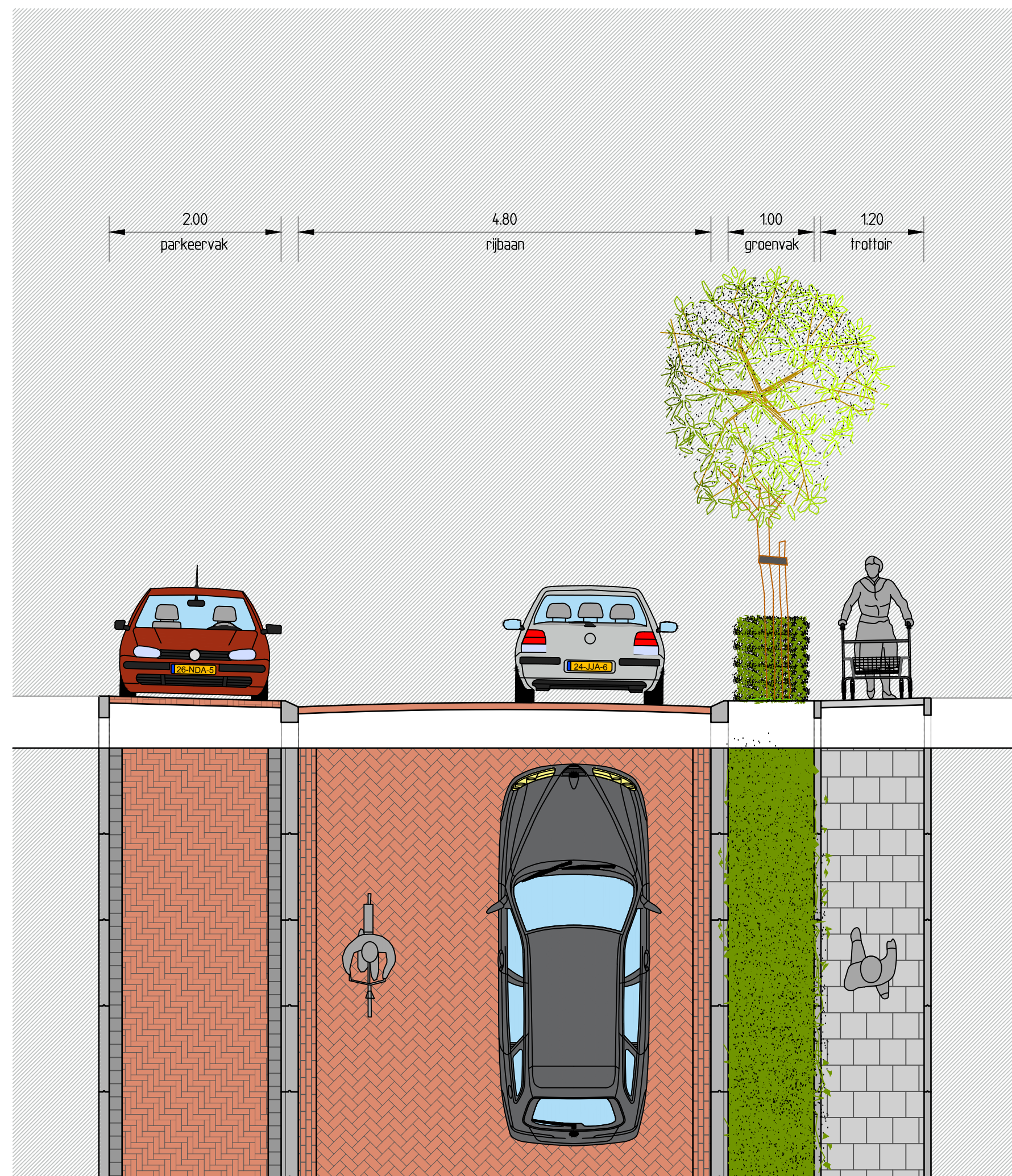
Dwarsprofiel C-C schaal: 1 : 50
