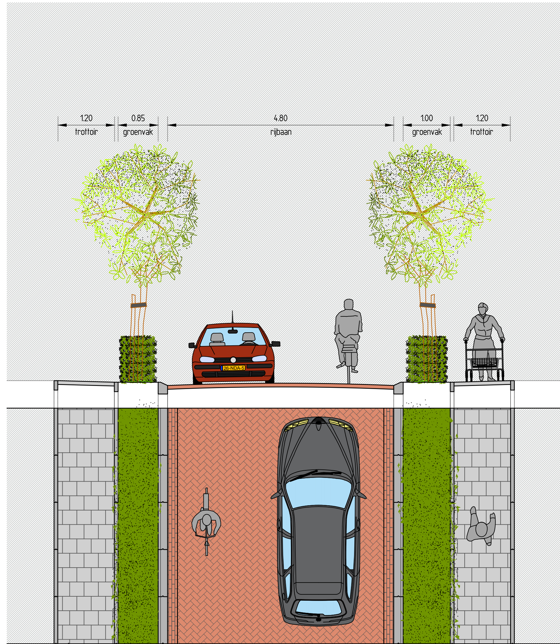
Dwarsprofiel D-D schaal: 1 : 50
