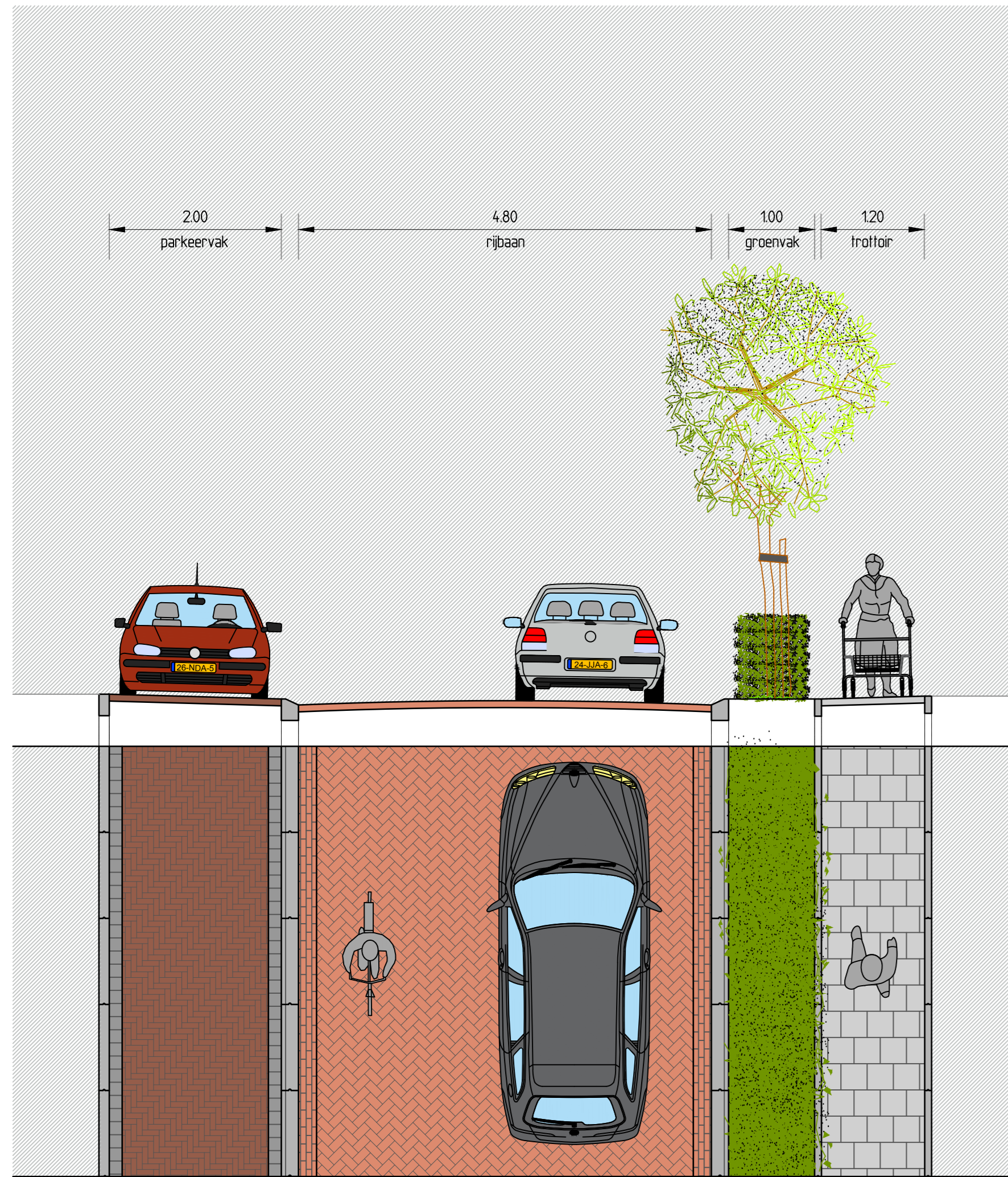
Dwarsprofiel C-C schaal: 1 : 50
